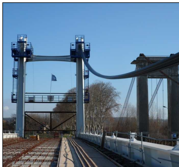
Vue d'ensemble avec le câble côté amont
